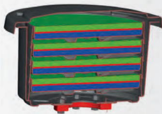
Mehrfachkammer-Filter
